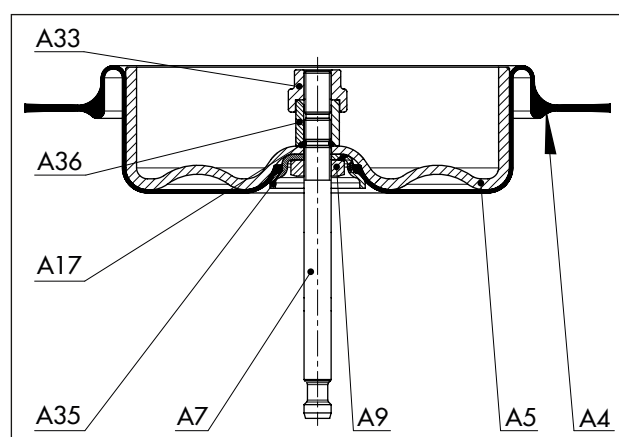
图 23: 针对“推杆伸出”动作方向 (175v2 和 350v2 cm 2 ) 的部件排列
