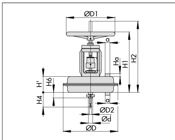
图 5: 3271 型, 带额外手轮
