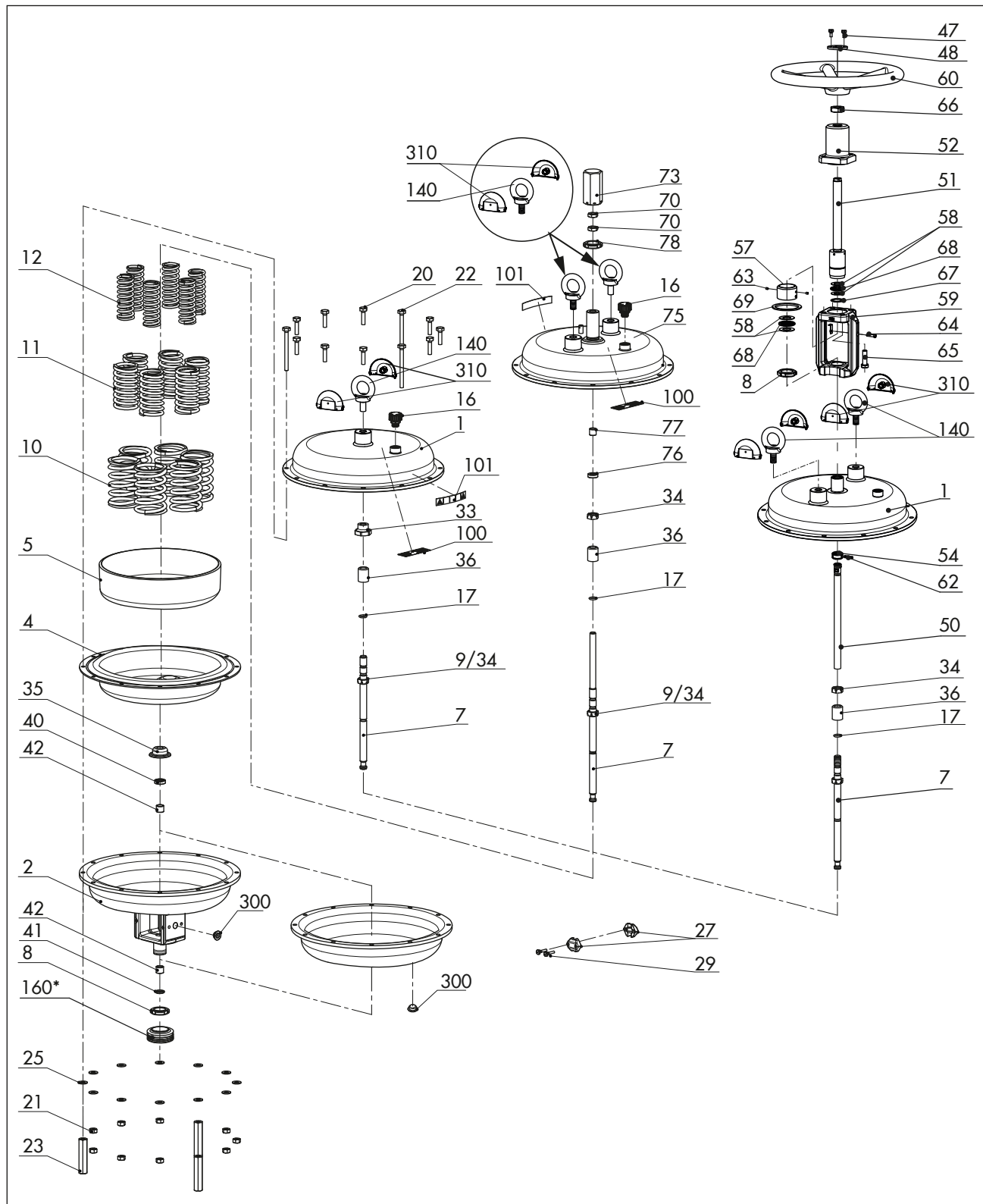
图 33: 3271/3277 型执行机构 (175v2/350v2/750v2 cm 2 )
