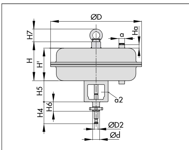
图 8: 3277 型, 所附支架用于直接连接附件 · 750v2 cm 2 执行机构面积
