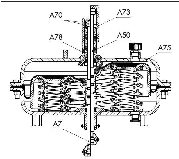
图 20: 带行程限位的 3271 型执行机构 (750v2 cm 2 , 带“推杆缩回”)
