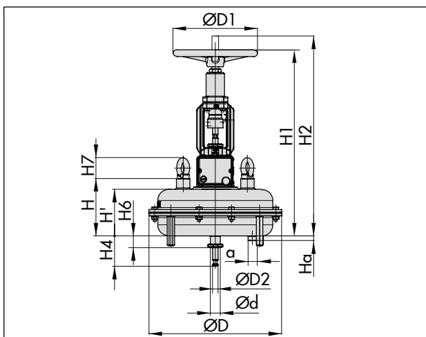
图 6: 两侧带手轮和行程限位的 3271 型气动执行机构
