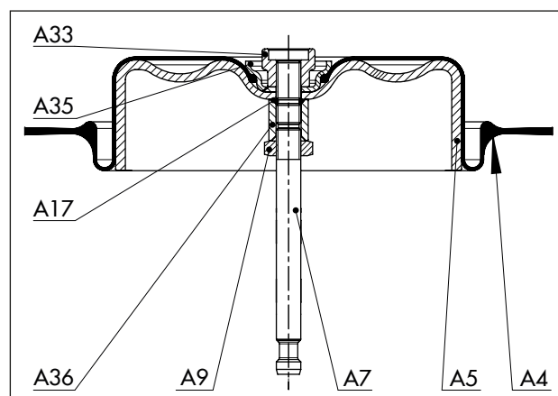
图 28: 针对“推杆缩回”动作方向 (175v2 和 350v2 cm 2 ) 的部件排列
