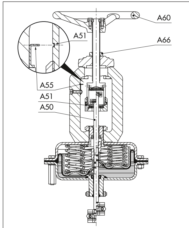
图 21: 带手轮的 3271 型执行机构 (175v2 或 350v2 cm 2 )
