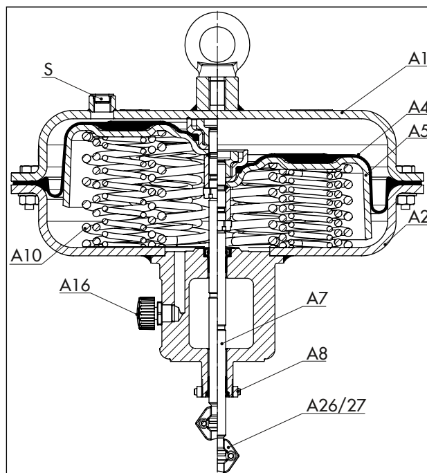
图 3: 3277 型执行机构，显示了 750v2 cm 2 执行机构面积以及“推杆缩回”动作方向的示例绘图
