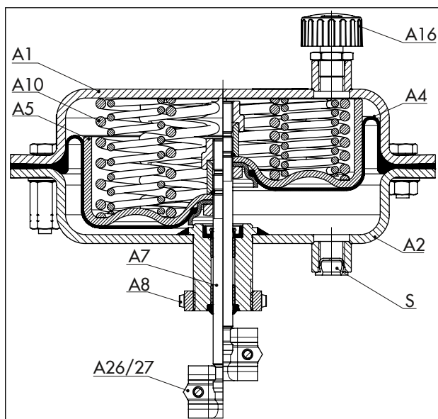
图 2: 3271 型执行机构，显示了 175v2 cm 2 执行机构面各以及“推杆伸出”动作方向的示例绘图
