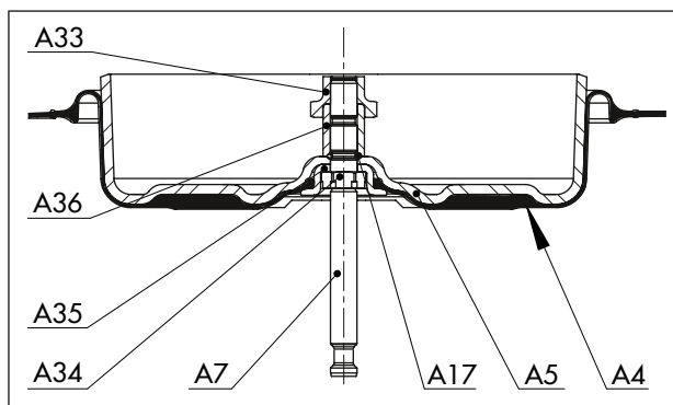
图 31: 针对“推杆伸出”动作方向 (750v2 cm 2 ) 的部件排列
