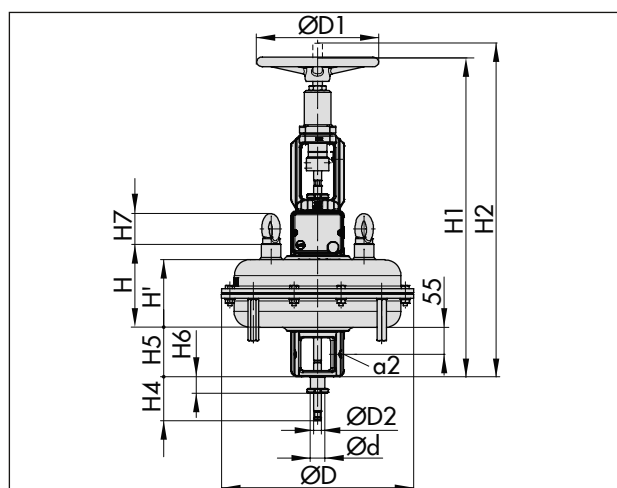
图 11: 两侧带手轮和行程限位的 3277 型气动执行机构
