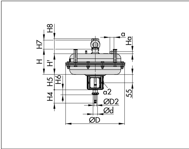
图 12: 3277 型, 带行程限位
