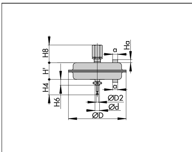
图 7: 3271 型, 带行程限位
