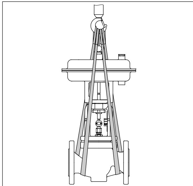
图 15: 控制阀上的吊点（所示示例）
