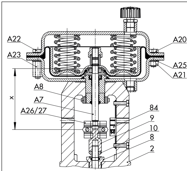
图 16: 单座直通阀上安装的 3271 型气动执行机构
