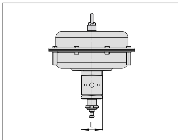
图 9: 带支架的 3277 型 (侧视图) · 750v2 cm 2 执行机构面积
