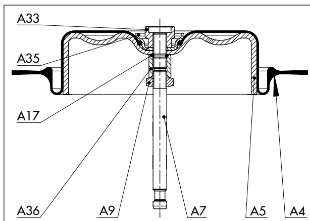
图 25: 针对“推杆缩回”动作方向 (175v2 和 350v2 cm 2 ) 的部件排列
