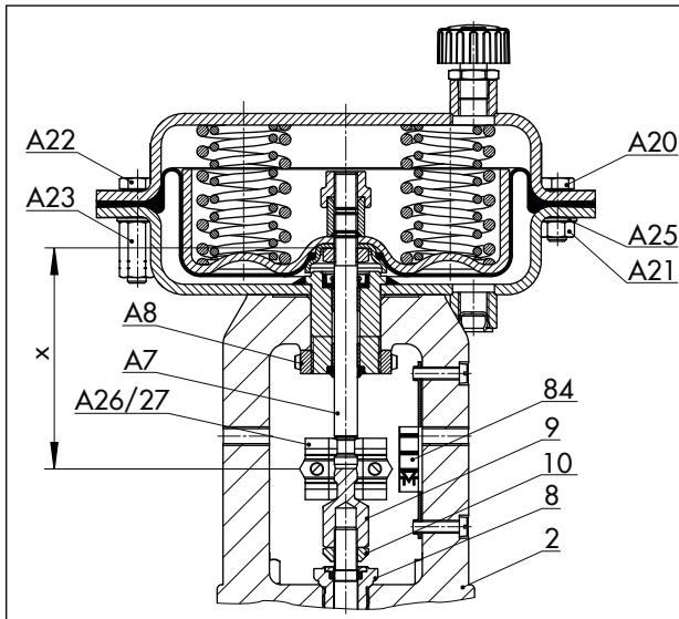
图 18: 单座直通阀上安装的 3271 型气动执行机构
