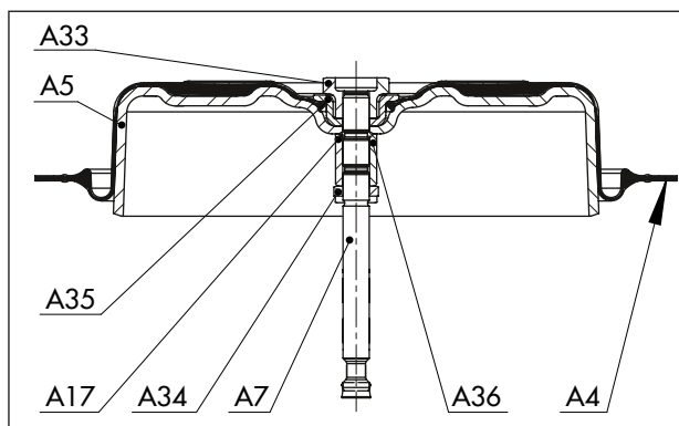
图 26: 针对“推杆缩回”动作方向 (750v2 cm 2 ) 的部件排列
