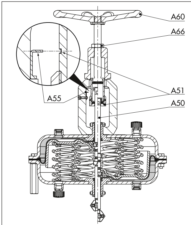
图 22: 带手轮的 3271 型执行机构 (750v2 cm 2 )
