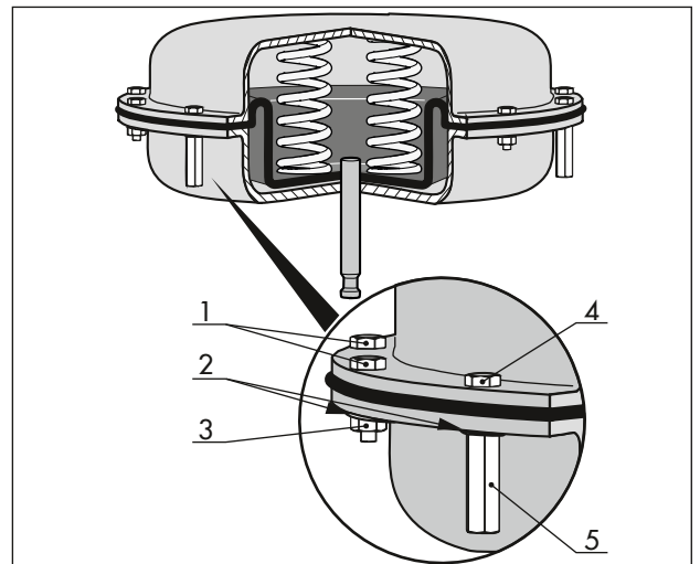
图 32: 预加载弹簧 (功能图)
