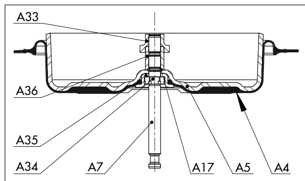
图 24: 针对“推杆伸出”动作方向 (750v2 cm 2 ) 的部件排列
