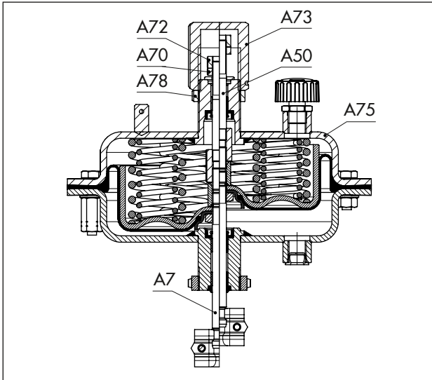
图 19: 带行程限位的 3271 型执行机构 (175v2 或 350v2 cm 2 , 带“推杆伸出”)
