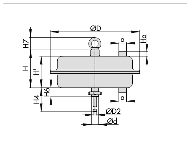
图 4: 执行机构面积为 750v2 cm 2 的 3271 型
