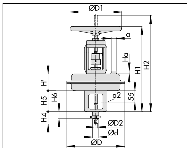
图 10: 3277 型, 带额外手轮
